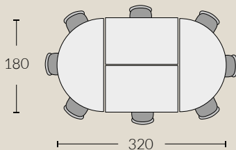
K-4T.ML.F+8SD.ST.D180320
